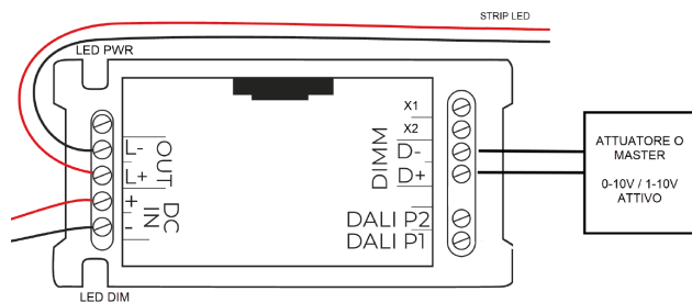
COLLEGAMENTO 0-10V PHASE-CUT-CV - FIGURA N. 3
