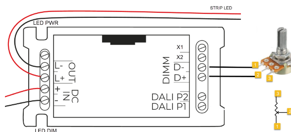
COLLEGAMENTO POTENZIOMETRO PHASE-CUT-CV-UL - FIGURA N. 2
