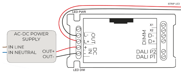
SCHEMA COLLEGAMENTO ALIMENTAZIONE E LED PHASE-CUT-CV-UL - FIGURA N. 1
