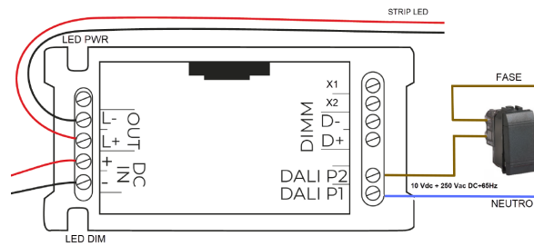
COLLEGAMENTO PULSANTE PHASE-CUT-CV - FIGURA N. 4
